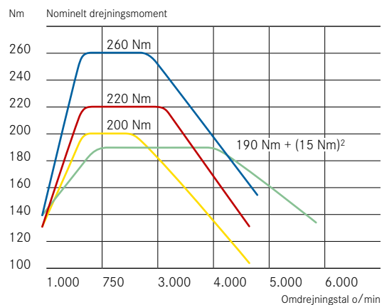
Momentkurver:
